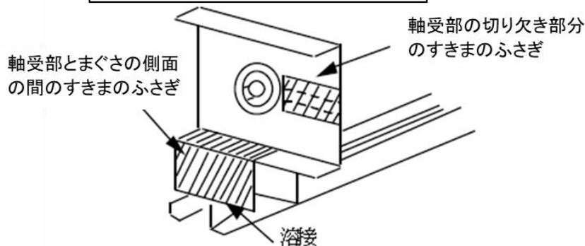
軸受部とまぐさの側面の間及び軸受部の切り欠き部分のすきまのふさぎ(例)
