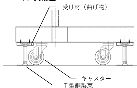
A 矢視図
